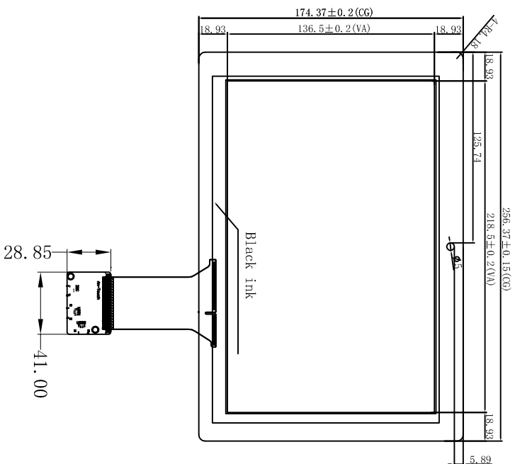
正视图
