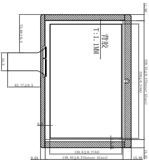
背视图
