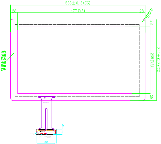
正视图
